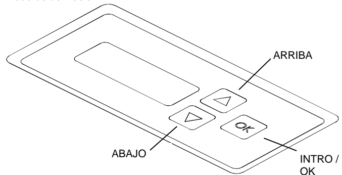
Esquema de la interfaz de usuario LCD del equipo eWire™ Pro
